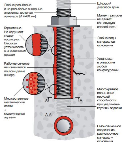
Химический анкер BIT
