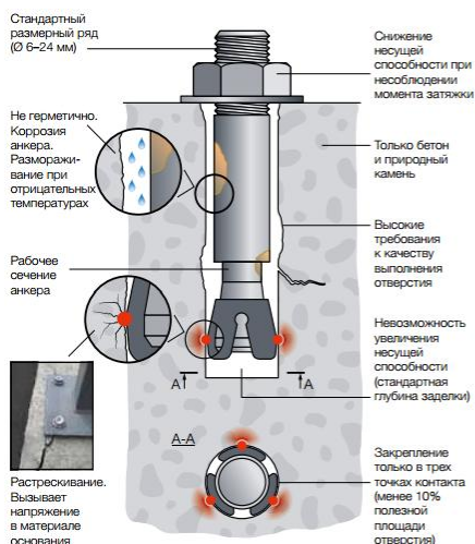
Распорный металлический анкер
