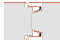
УЗЕЛ СОЕДИНЕНИЯ ПАНЕЛЕЙ
