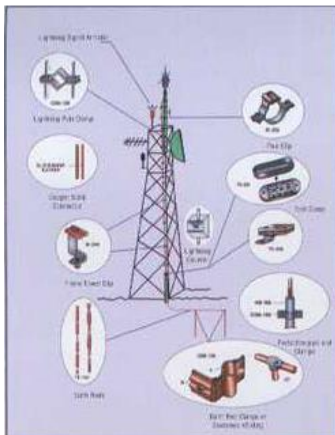
Фрагмент монтажа опоры молниезащитного устройства от земли.
